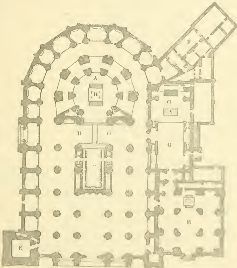
Abbild. 2 Kathedrale von Granada. Grundriß. A Capilla mayor, B Altar, C Chor, D Querschiff, E Glockenthurm, F Sakristei, G Capilla Real, H Sagrario, an der Stelle der alten Mariä hee.
